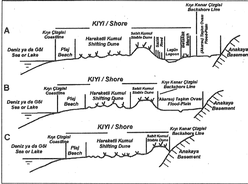
Türkiye'nin Akdeniz Kıyı kuşağındaki alçak kıyılarda yer alan kıyı şekilleri ve "Kıyı Kenar Çizgisi"ni sınırladığını gösteren şematik profiller (Özner, 1997'den).
